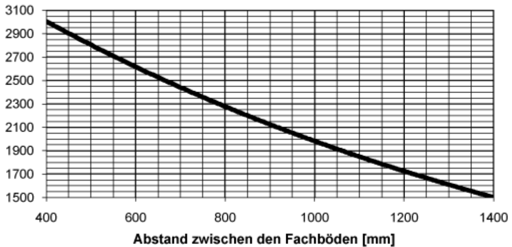
Tragkraft-Diagramm der Regalständer
