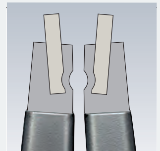
Formschluss durch Verpressung
