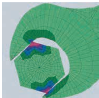
Herkömmlicher Schraubenschlüssel: Kantenpressung führt zu Beschädigung
